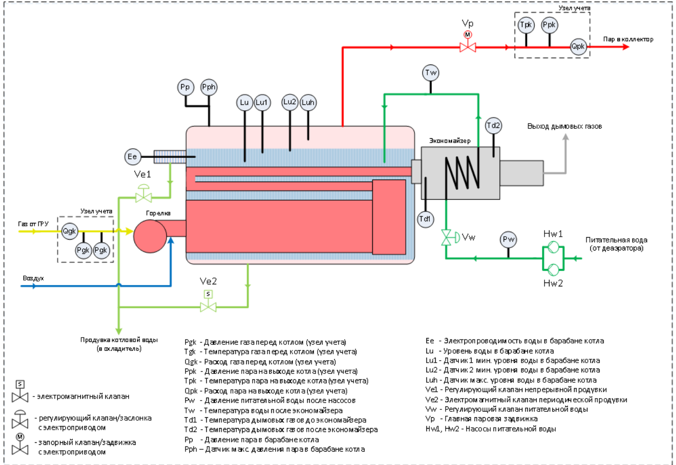
Типовая схема автоматизации парового котла с автоматизированной горелкой
